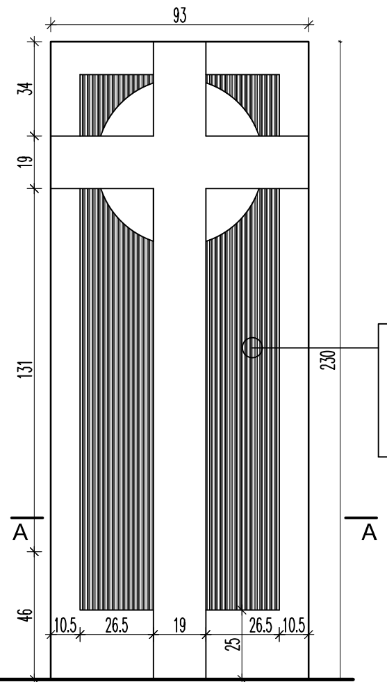
Widok drzwi do zakrystii skala 1:10
