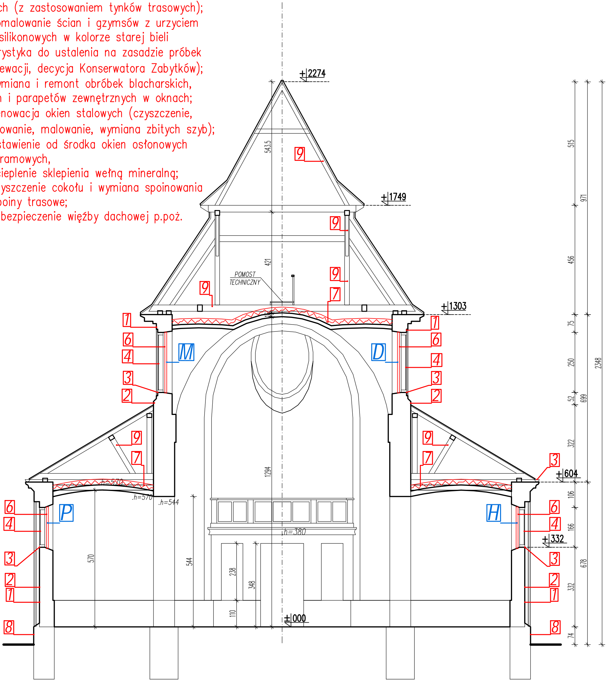
PRZEKRÓJ A-A
