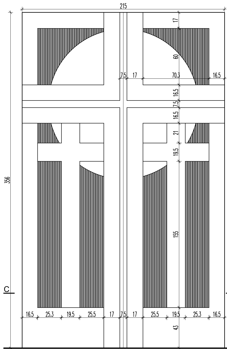
Widok drzwi głównych skala 1:10 Przekrój C-C przez fronton drzwi głównych skala 1:10
