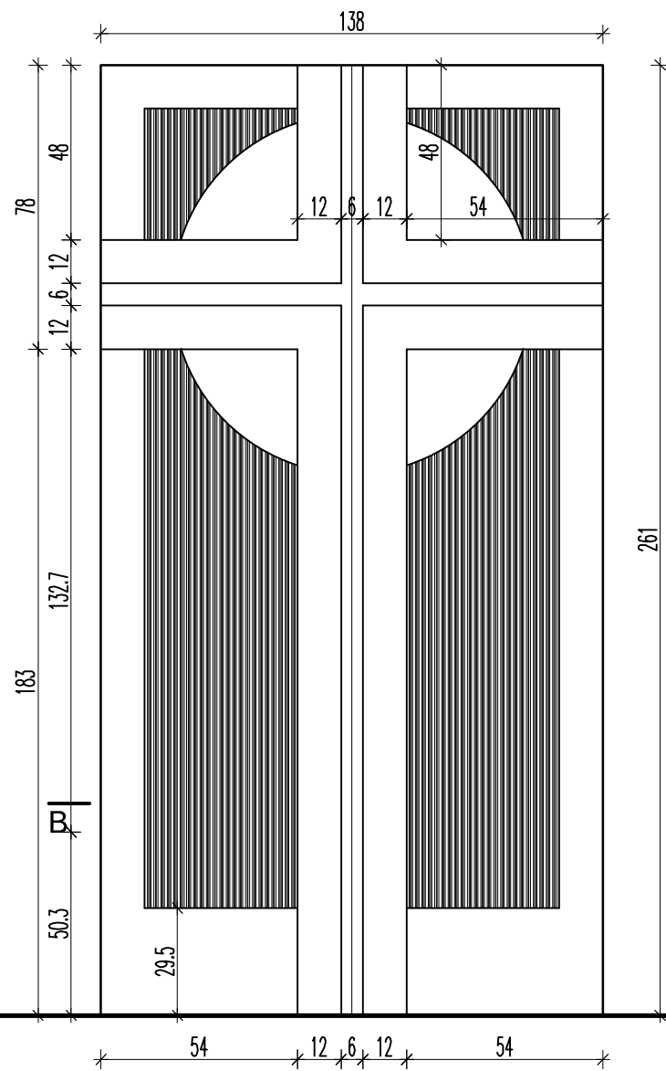
Widok drzwi bocznych skala 1:10
